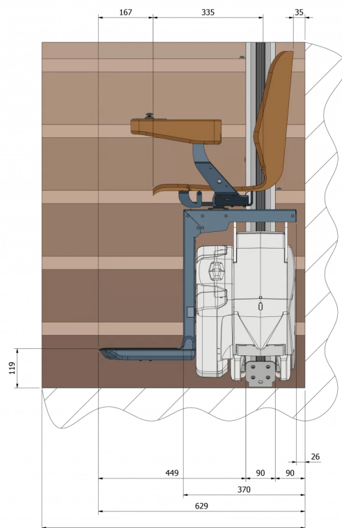
Largura mínima da escada 740mm
